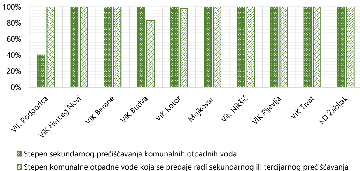
Grafik I.3.2.2 Poređenje vrijednosti Stepena komunalne otpadne vode koja se predaje radi sekundarnog ili tercijarnog prečišćavanja i Stepena sekundarnog prečišćavanja komunalnih otpadnih voda u 2025. godini [%]
