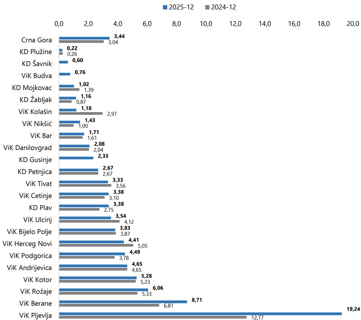
Grafik I.1.6.1 Poređenje vrijednosti Broja kvarova po kilometru vodovodne mreže po vršiocu sa vrijednostima 2025. i 2024. godini [# / km]
