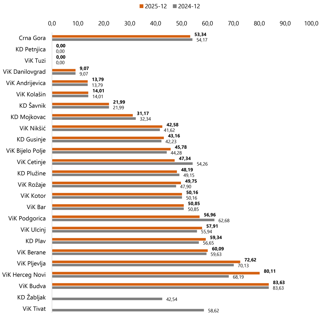
Grafik I.2.1.2 Poređenje vrijednosti Stepena pokrivenosti stanovništva uslugom putem priključaka na javni kanalizacioni sistem po vršiocu sa vrijednostima za 2025. i 2024. godinu [%]
