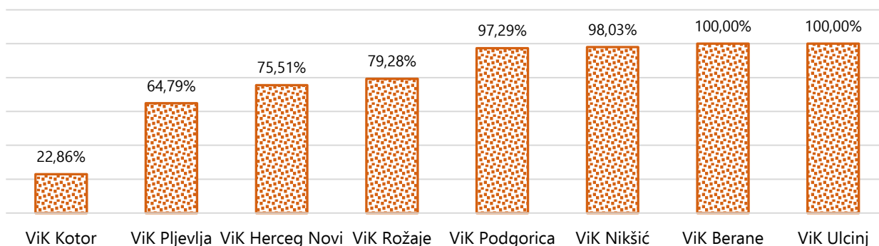
Grafik I.2.3.2 Poređenje vrijednosti stepena pregledane kanalizacione mreže po vršiocu za 2025. i 2024. godinu [%]
