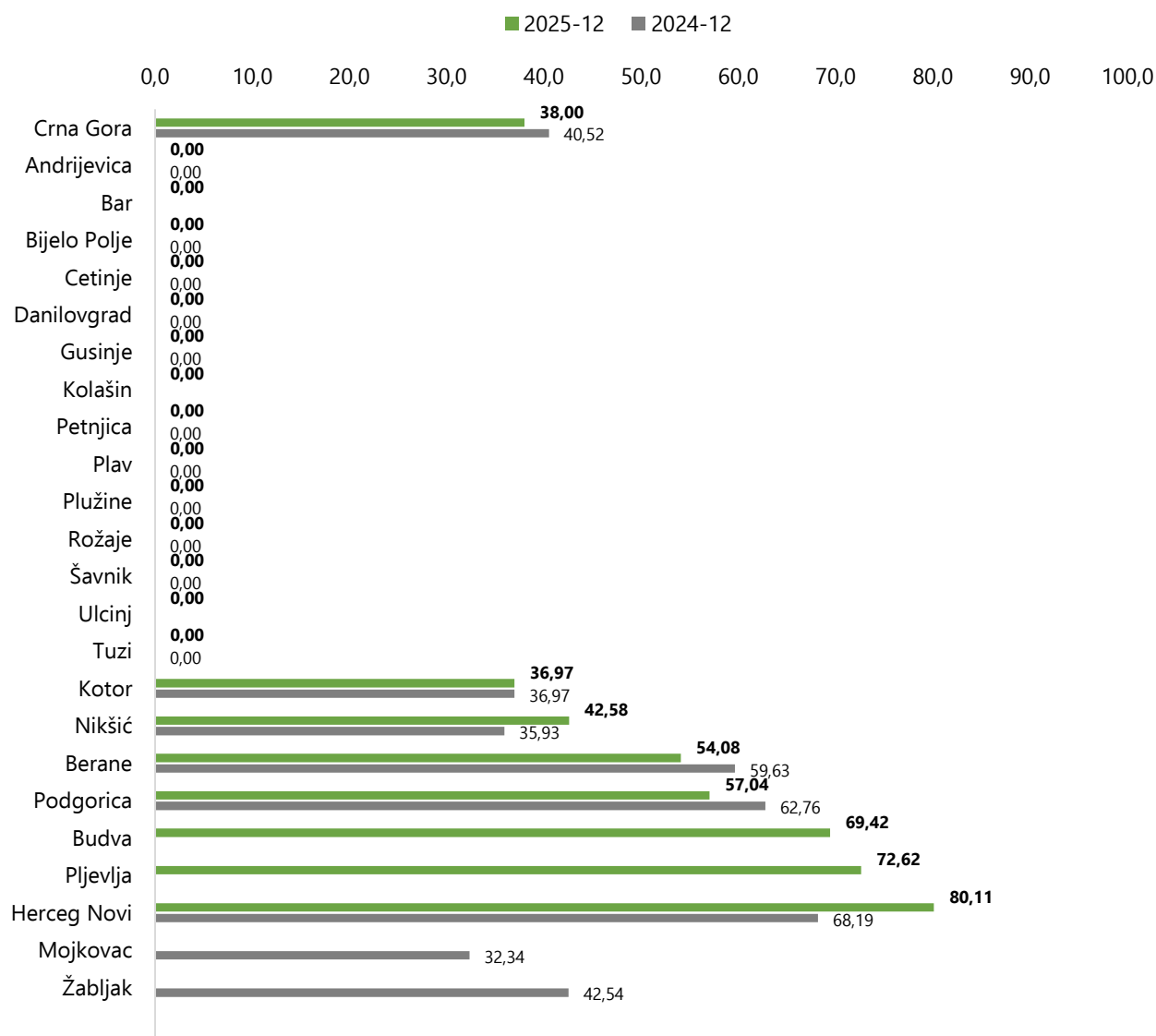
Grafik 1.3.3.1 Poređenje vrijednosti stepena pokrivenosti stanovništva uslugom prečišćavanja komunalnih otpadnih voda po vršiocu sa vrijednostima za 2025. i 2024. godinu [%]
