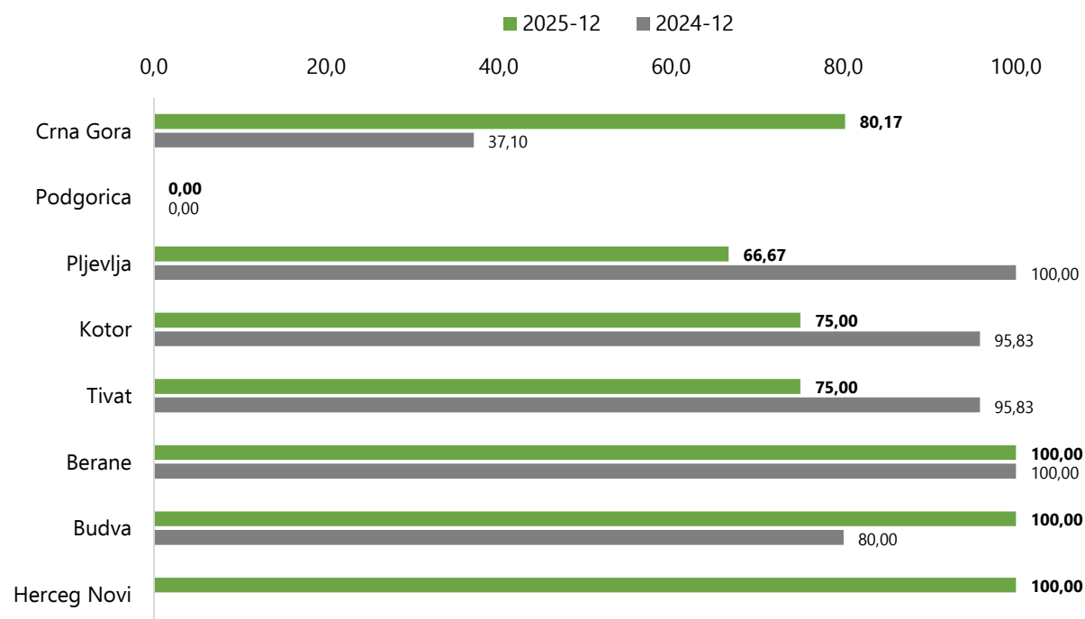
Grafik I.3.1.1 Poređenje vrijednosti Stepena usaglašenosti kvaliteta efluenta po vršiocu sa vrijednostima za 2025. i 2024. godinu [%]
