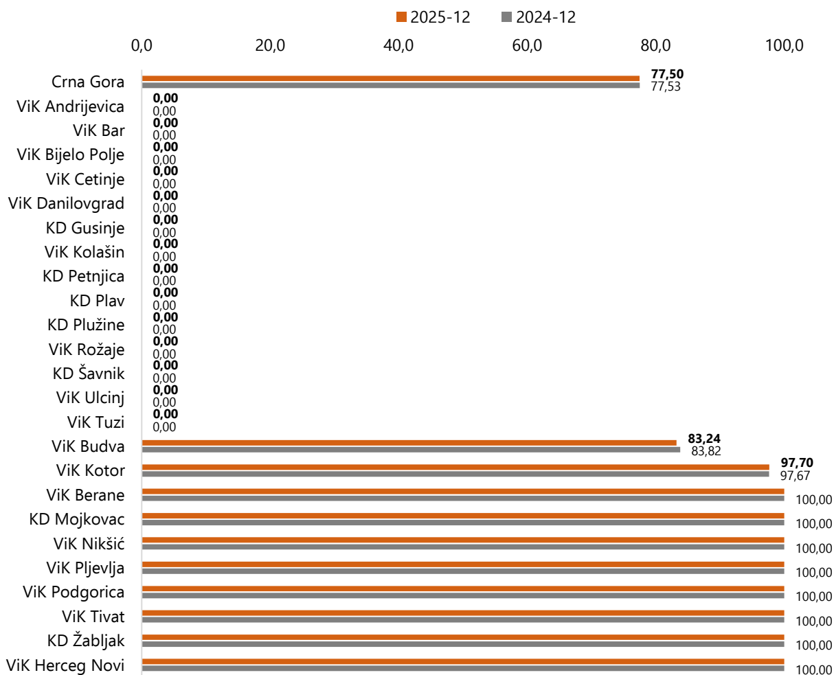
Grafik I.2.2.1 Poređenje vrijednosti Stepena komunalne otpadne vode koja se predaje radi sekundarnog ili tercijarnog prečišćavanja po vršiocu sa vrijednostima za 2025. i 2024. godinu [%]
