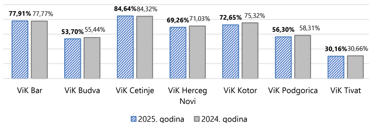
Grafik I.1.4.3 Poređenje vrijednosti neprihodovane vode po korisniku mjesečno za vršioce koji mjere zahvaćene i veći dio količine fakturisane vode za 2025. i 2024. godinu [m 3 /korisnik / mjesec]
