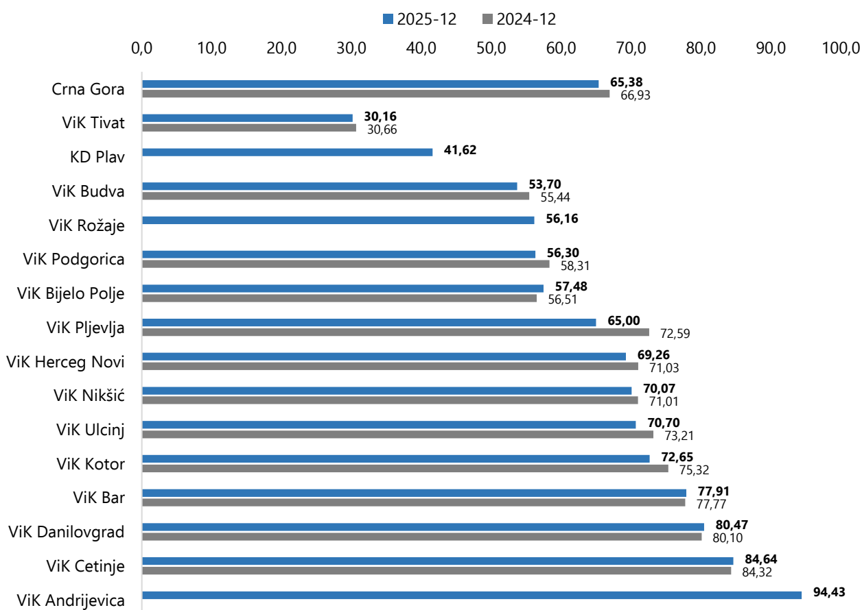
Grafik I.1.4.2 Poređenje vrijednosti stepena neprihodovane vode po vršiocu za 2025. i 2024. godinu [%]
