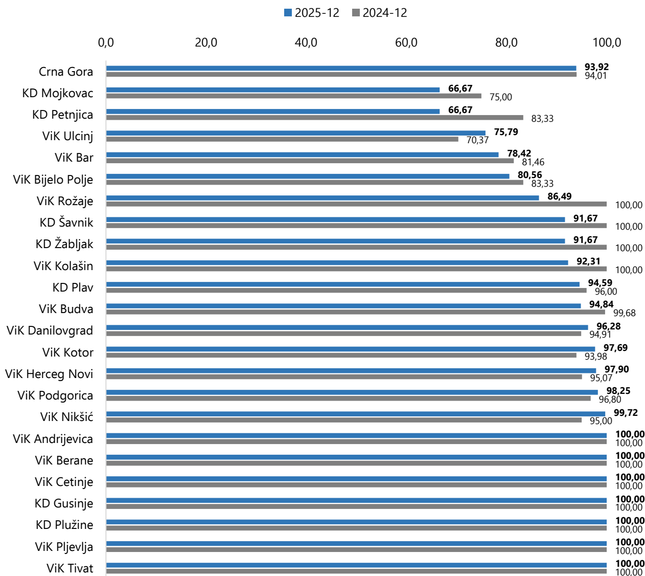
Grafik I.1.2.1 Poređenje vrijednosti stepena usaglašenosti kvaliteta vode sa posebnim propisima po vršiocu za 2025. i 2024. godinu [%]
