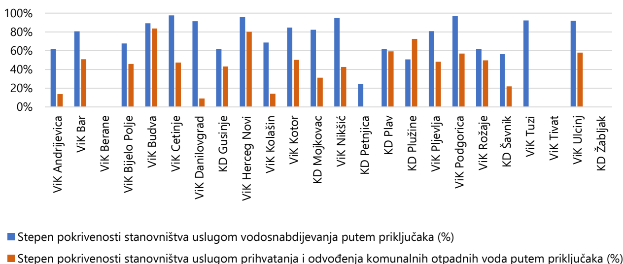
Grafik I.2.1.1 Poređenje vrijednosti Stepena pokrivenosti stanovništva uslugom vodosnabdijevanja putem priključaka i Stepena pokrivenosti stanovništva uslugom prihvatanja i odvođenja komunalnih otpadnih voda putem priključaka na javni kanalizacioni sistem po vršiocu u 2025. godini [%]
