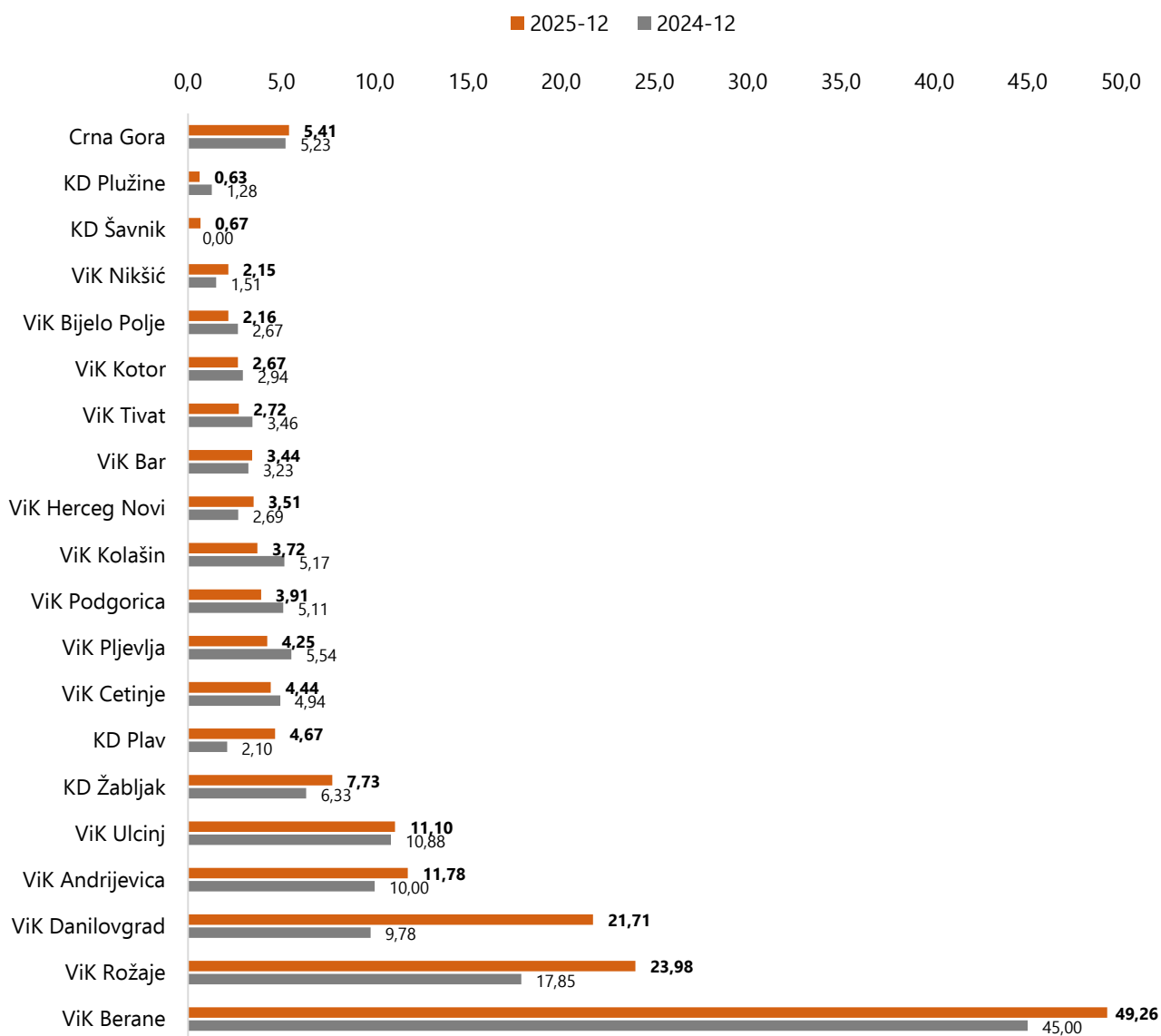
Grafik I.2.4.1 Poređenje vrijednosti broja začepljenja po kilometru kanalizacione mreže po vršiocu sa vrijednostima za 2025. i 2024. godinu [# / km]
